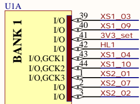
XC9572XL-10VQG44C
